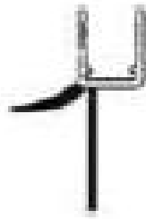
AC6845091-2 ACTIV LIPPENDICHTUNG 30MM MIT WASSERABWEISER 135° FÜR 6-8MM GLAS LÄNGE 2010MM
